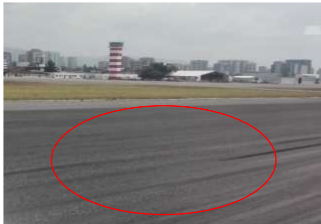
Imagen 7.4.2 Pérdida del Agregado fino de la pista
